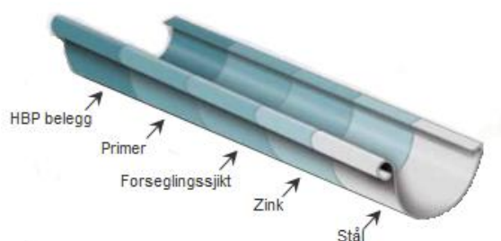
Figur 1 oppbygging av takrenne
