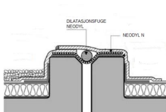
Figur 1, eksempel på ekspansjonsfuge
