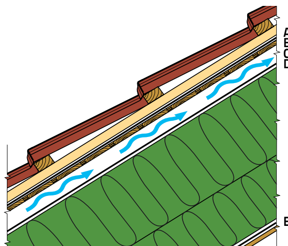
Ultra D underlagsbelegg [A] Bærende taktro [B] Luftespalte [C] Vindsperre [D] Dampsperre [E]
